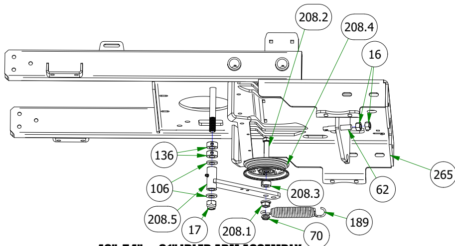
48", 54", & 61" IDLER ARM ASSEMBLY
