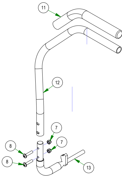
031-8851-70 ZT Steering Arm - Right
