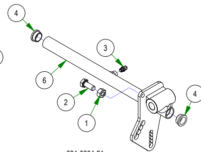
031-0054-21 2021 Maverick Drive Arm Actuator LH Assembly
